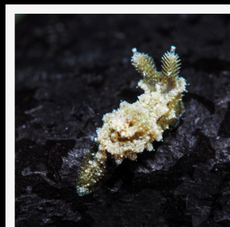
Polycera herthae
