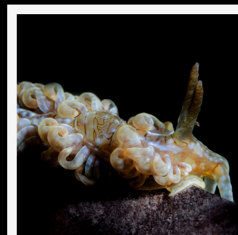
Spurilla dupontae
