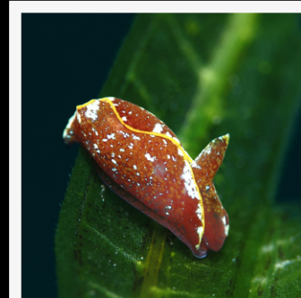
Gastropteron chacmol
